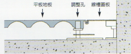
收邊剖面示意圖
