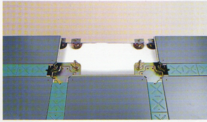
面板收邊處理(可現場裁切)
