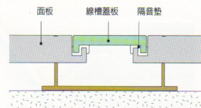
線槽蓋與面板採嵌入式設計，穩定性高，防震效果佳。
